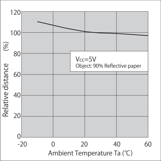
検出距離特性－周囲温度特性 (代表例) Relative distance vs. Ambient Temperature (typ.)
