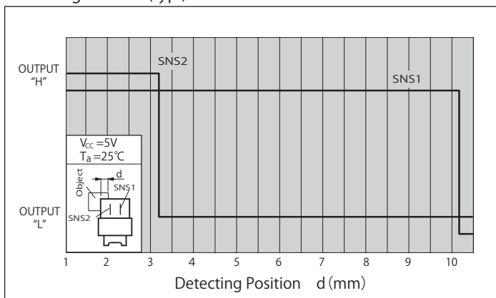
検出位置特性1 (代表例) Detecting Position (typ.)
