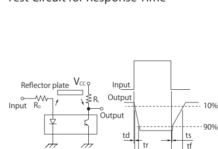
応答時間測定回路
