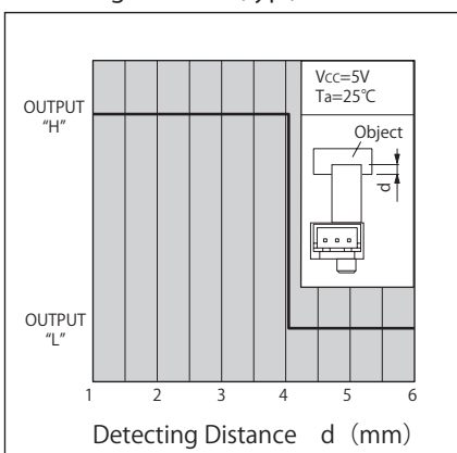
検出位置特性2 (代表例) KI3051/3053
