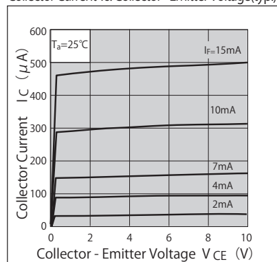
光電流-コレクタエミッタ間電圧特性 (代表例) Collector Current vs. Collector - Emitter Voltage (typ.)
