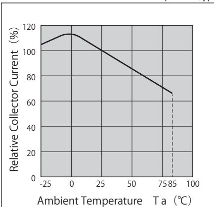
相対光電流－周囲温度特性 (代表例) Relative Collector Current vs. Ambient Temperature (typ.)
