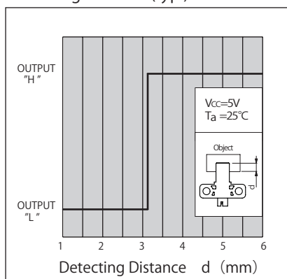
検出位置特性2 (代表例) KI5351 Detecting Distance (typ.)
