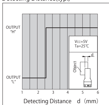
検出位置特性1 (代表例) KI3111 Detecting Distance (typ.)
