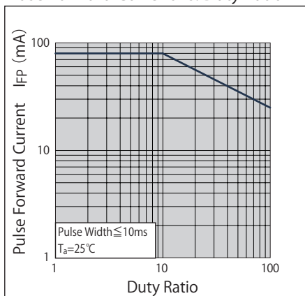
パルス順電流—デューティ比 Pulse Forward Current vs. Duty Ratio
