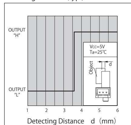
検出位置特性1 (代表例) KI3051/3053
