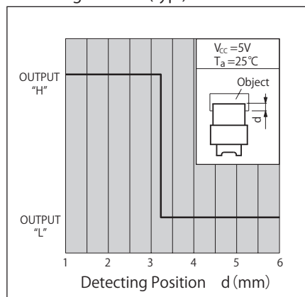
検出位置特性2 (代表例) Detecting Position (typ.)
