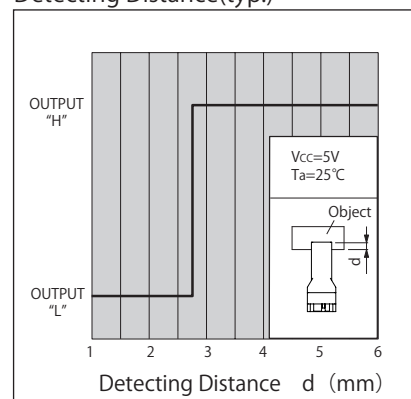
検出位置特性2 (代表例) KI3111 Detecting Distance (typ.)
