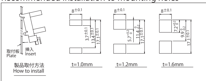
推奨取付穴寸法図
