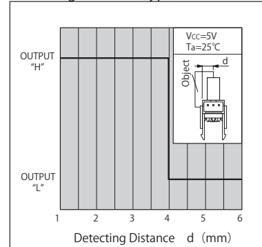
検出位置特性 2 (代表例) KI1306
