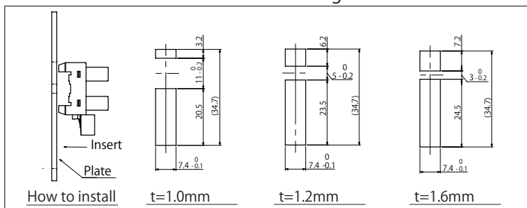
推奨取付穴寸法図
