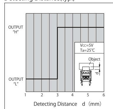
検出位置特性2 (代表特性) KI3781 Detecting Distance (typ.)
