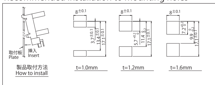
推奨取付穴寸法図
