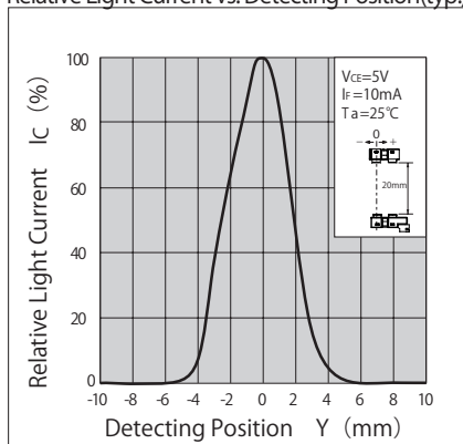
平行移動特性(代表例)
