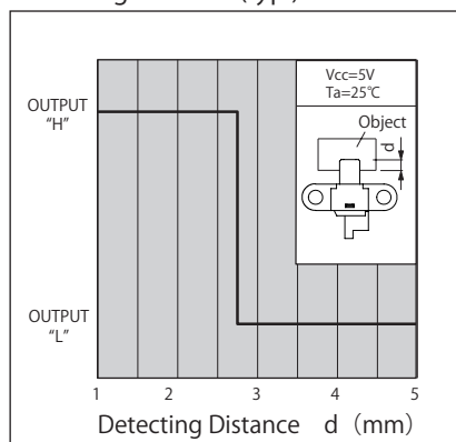
検出位置特性2 (代表例) KI5230 Detecting Distance (typ.)
