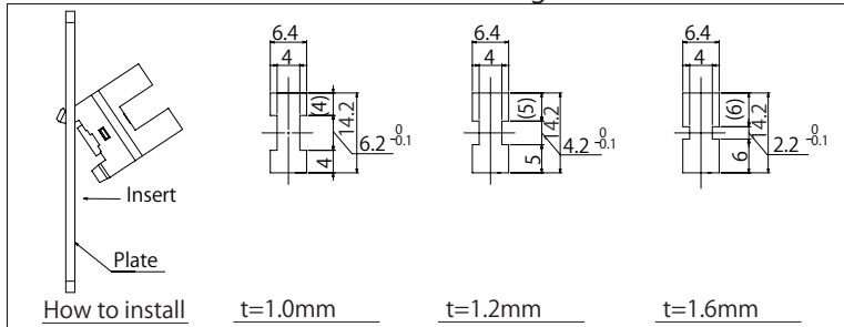
推奨取付穴寸法図
