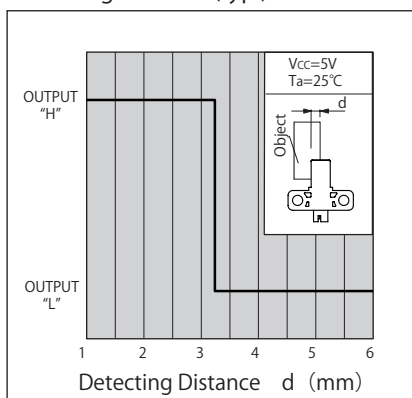
検出位置特性1 (代表例) KI5350 Detecting Distance (typ.)
