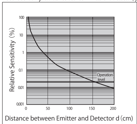
相対受光出力ー 設定距離特性(代表例) KB5921 ※2 Relative Sensitivity vs. Distance between Emitter and Detector (typ.)
