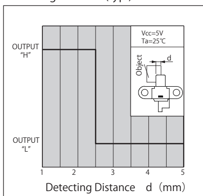
検出位置特性1 (代表例) KI5230 Detecting Distance (typ.)
