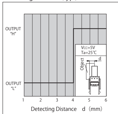
検出位置特性 1 (代表例) KI1306
