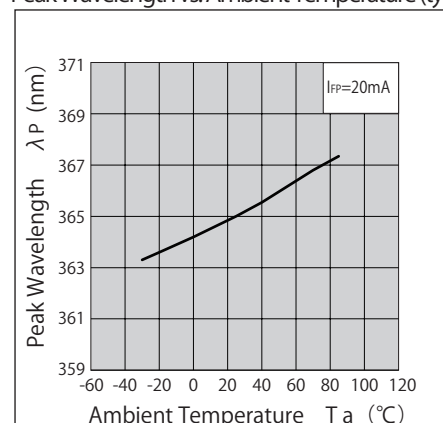
ピーク発光波長—周囲温度特性 (代表例) Peak Wavelength vs. Ambient Temperature (typ.)
