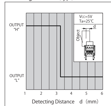
検出位置特性1 (代表特性) KI3780 Detecting Distance (typ.)
