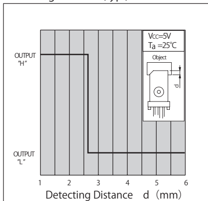
検出位置特性2(代表例) KI3990 Detecting Distance (typ.)
