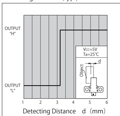
検出位置特性1 (代表例) KI5351 Detecting Distance (typ.)
