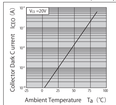
暗電流一周囲温度特性 (代表例)
