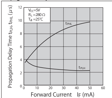
伝搬遅延時間一順電流特性 Propagation Delay Time vs. Forward Current
