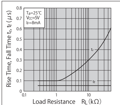
上昇・下降時間一負荷抵抗特性 Rise/Fall Time vs. Load Resistance
