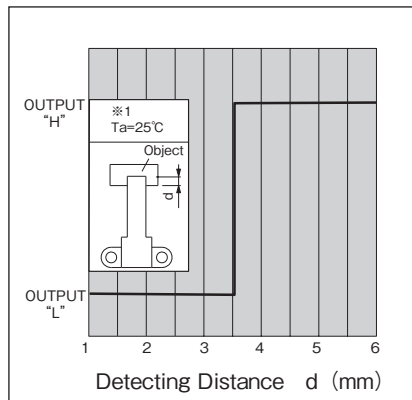
検出位置特性2 (代表例) KI3701/3710
