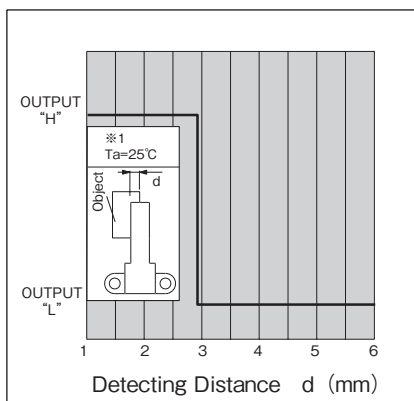
検出位置特性1 (代表例) KI3701/3710
