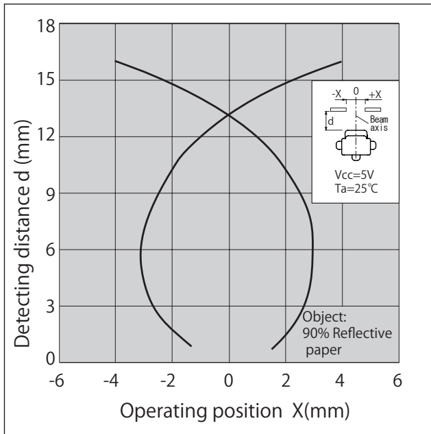
検出距離特性—動作位置1 (代表例)
