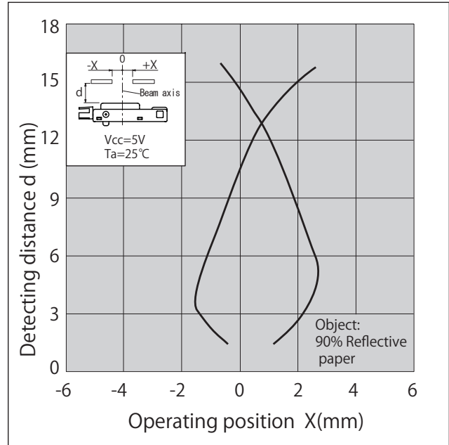
検出距離特性—動作位置2 (代表例)
