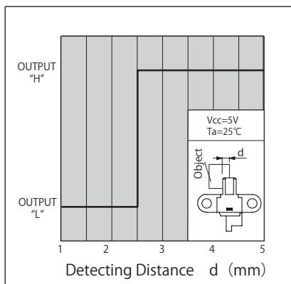
検出位置特性1 (代表例) KI3751
