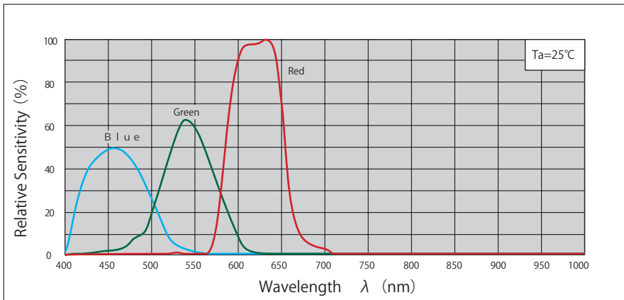
分光感度特性(代表例)
